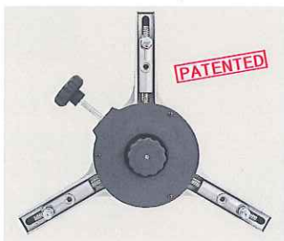
センタリングクランプ (8"~23"対応)
