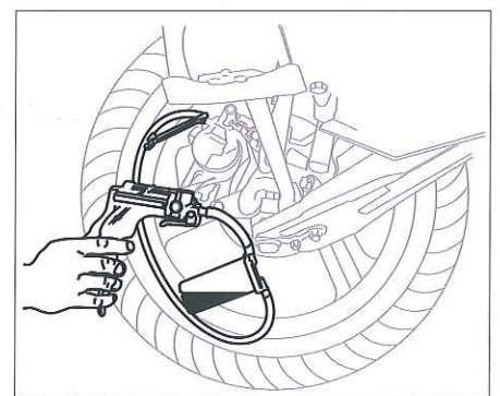
ブレーキフルードラインのエア抜き例
